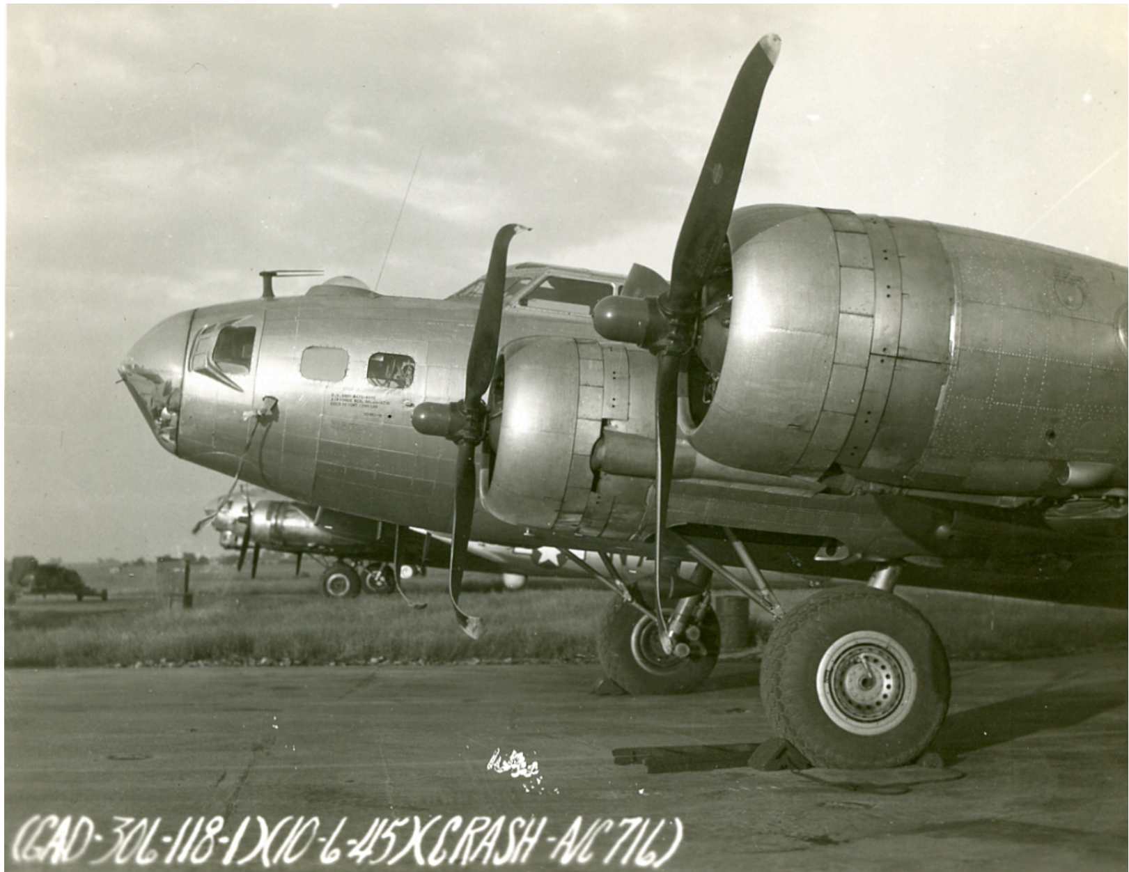
44-8716 model B-17G-80-VE
